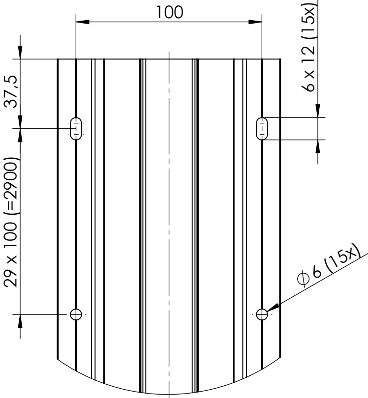
Detail Y 1:2
