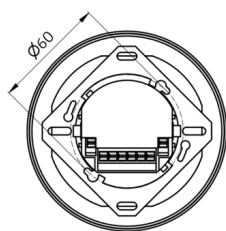
Bemaßung 92575
