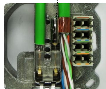
Abb.: Kabel auflegen
