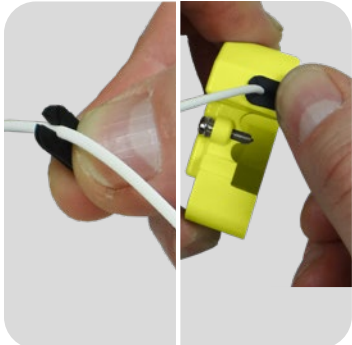
Abb.1-2: Klemmgummi an Kabel/Deckel anbringen
